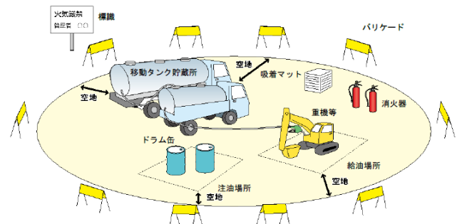
移動タンク貯蔵等による給油、注油等の安全対策の例
