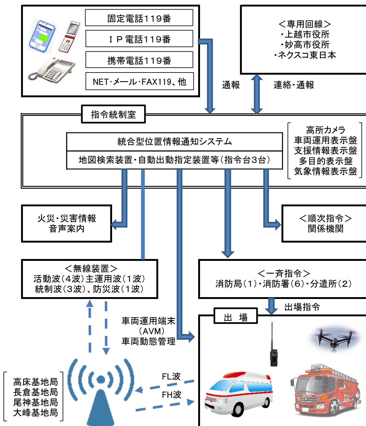
指令統制系統図
